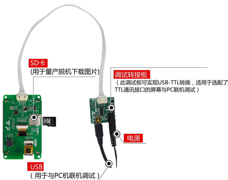
图 1-5 调试工具图
