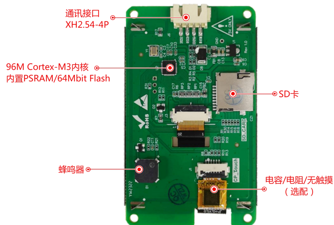
图 1-4 硬件配置图
